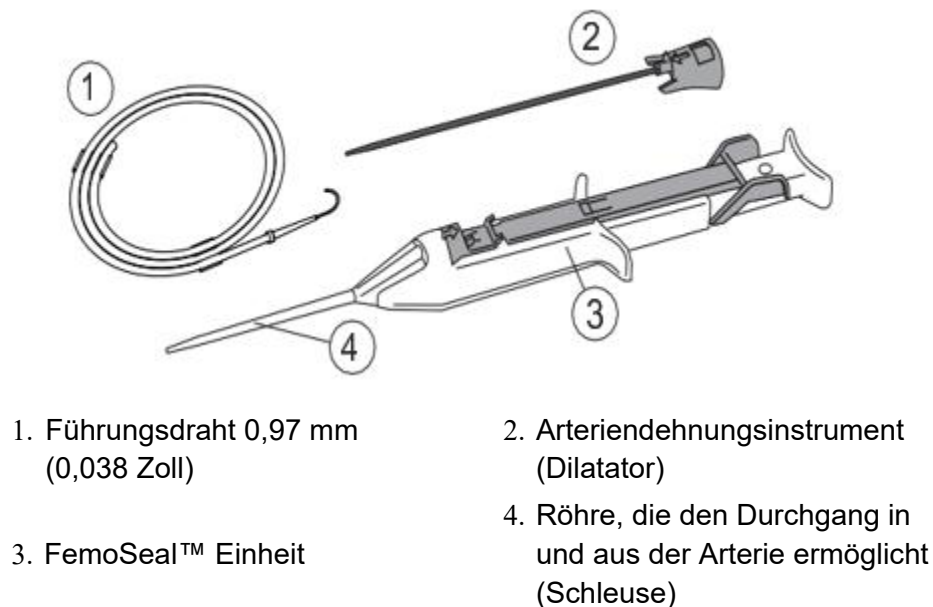
Abbildung 2.1 FemoSeal™ VCS Einheit mit Führungsdraht und Dilatator
