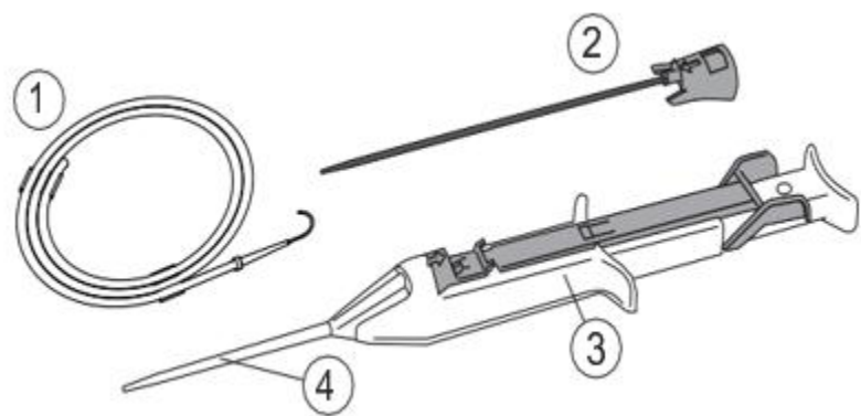
Figura 1.3 Unità FemoSeal™ VCS con filo guida e dilatatore
