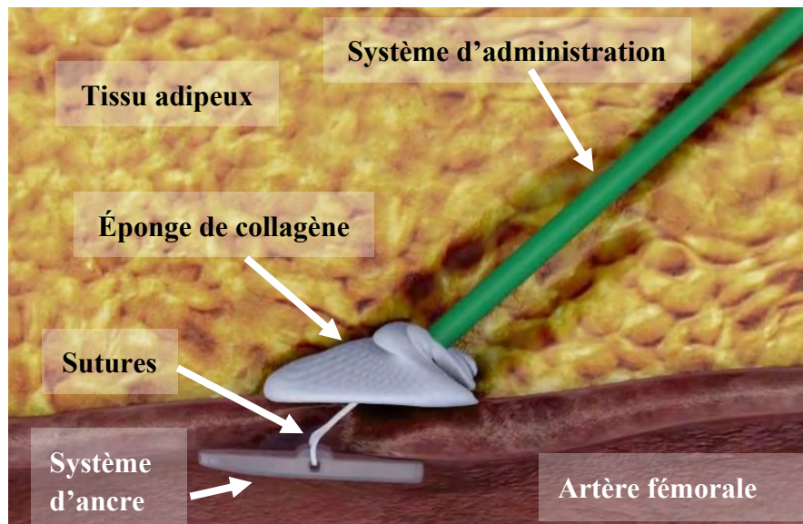
Schéma 1.1 Scellement de la ponction artérielle avec le Angio-Seal™ VIP VCD
